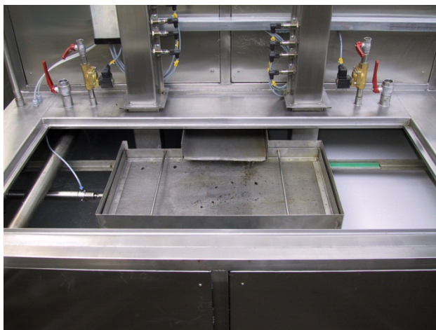
Rücklauf mit Filterkasten (hier 2-Bad-Anlage)
